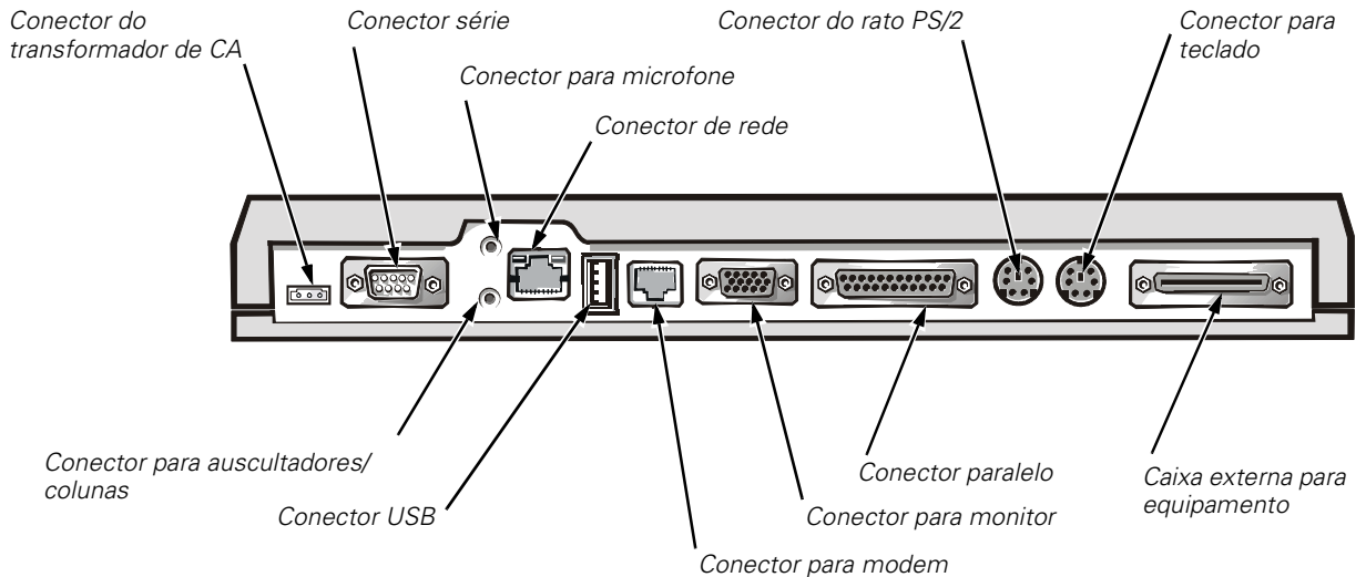
Figura 12-1. Montar dispositivos externos no APR
